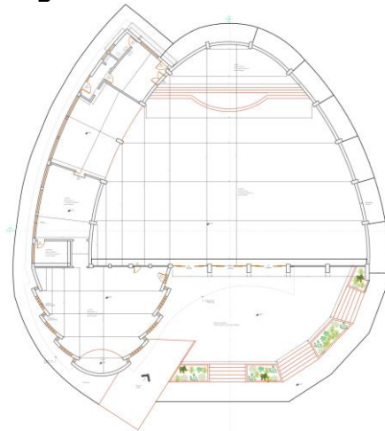
Imagem 06: Planta baixa técnica
